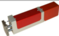
LH - Unité Linéaire Course 200 mm Piston 226 N à 5 bar Charge 275 N
