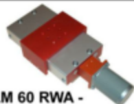
LM 60 RWA - Unité Linéaire Couverte Actionneur linéaire électrique Course 400 mm / Charge 750 N Rail double / Rattrapage de jeu Vis à billes pas 5 mm
