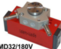
MD32/180V Unité rotative Rotation 180° Couple 3.6 Nm à 5 bars
